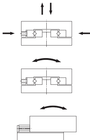
图2 负荷方向
